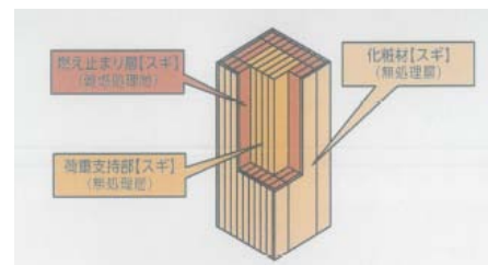
純木質耐火集成材(木ぐるみFR)断面概要 (※ご協力 住友林業)
